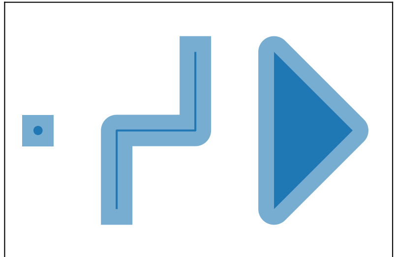
s.buffer(0.2, cap_style=3)
