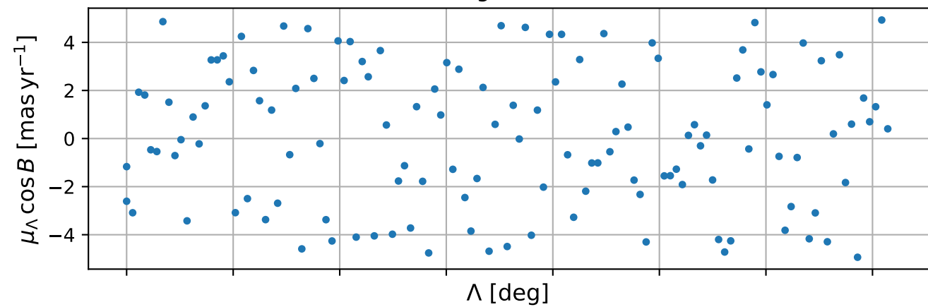
Sagittarius
